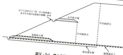
図 V・2-1 盛土の排水施設の概要図
