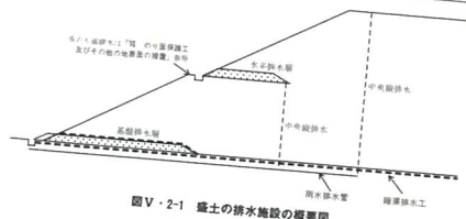
図 V-2-1 盛土の排水施設の概要図
