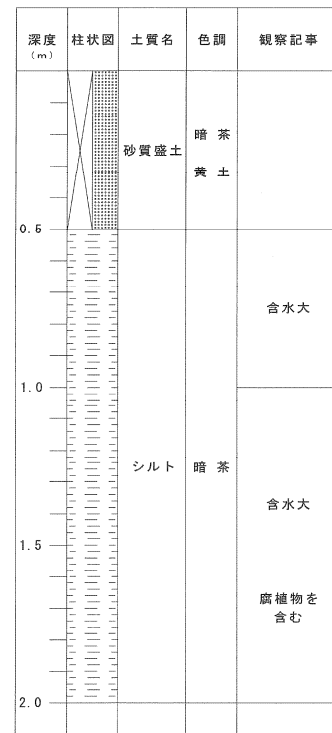
図-1 土質柱状図の例
